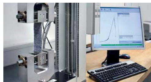
测定断裂强度和伸长率
