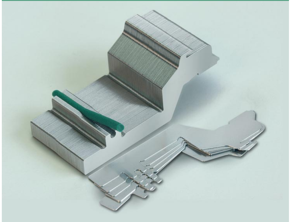
由象根带固定的沉降片
