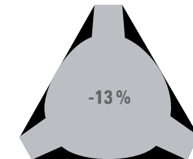
Vergleich des Querschnitts: Standard-Dreikant (außen) und EcoStar® (innen)
