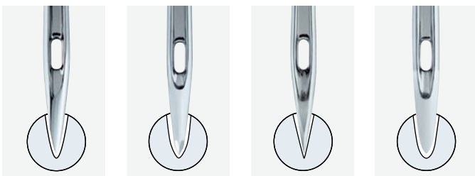
Beispiele verschiedener Schneidspitzen: LR, SD, P und S (von links)
